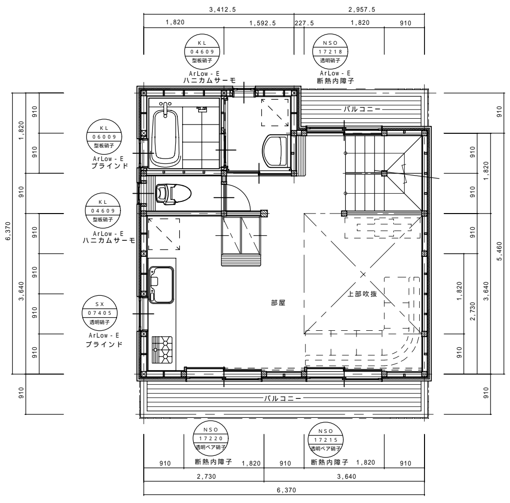
2 F 平面
