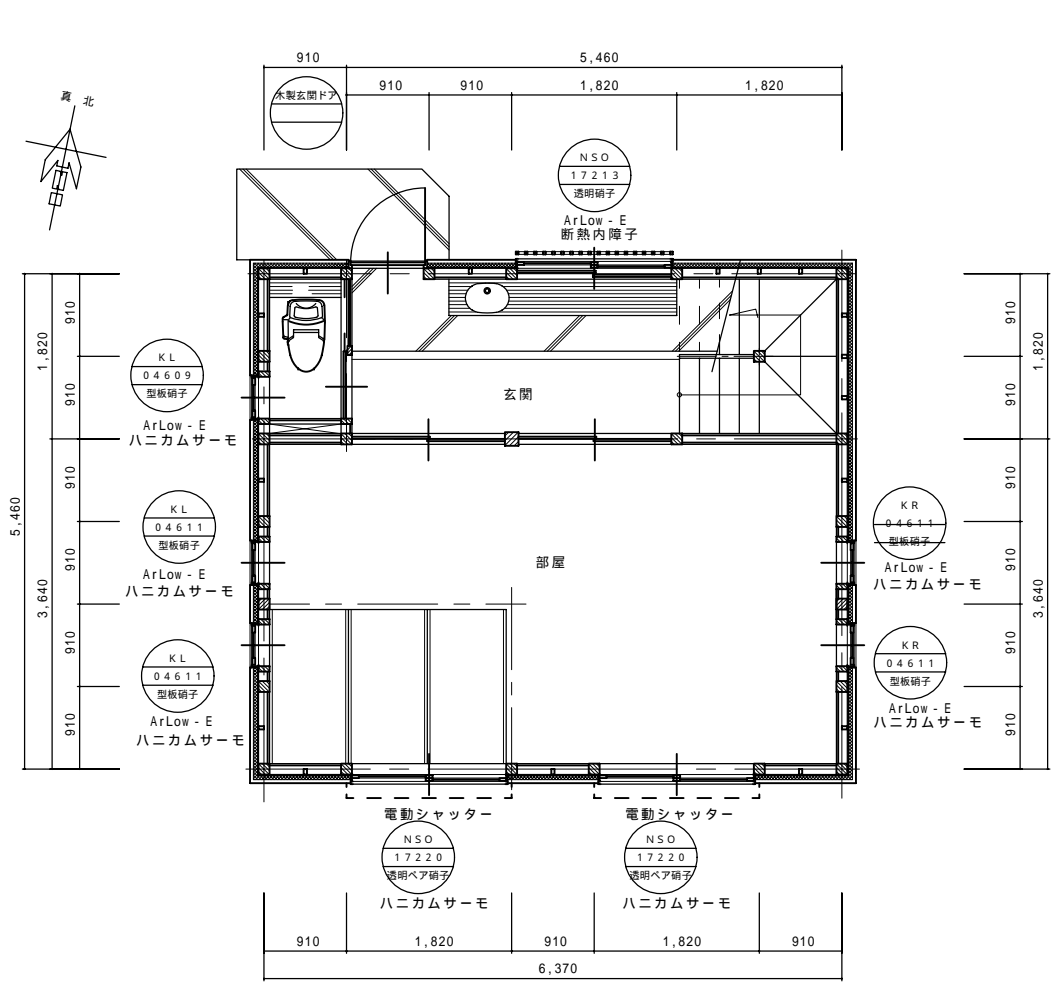
1 F 平面
