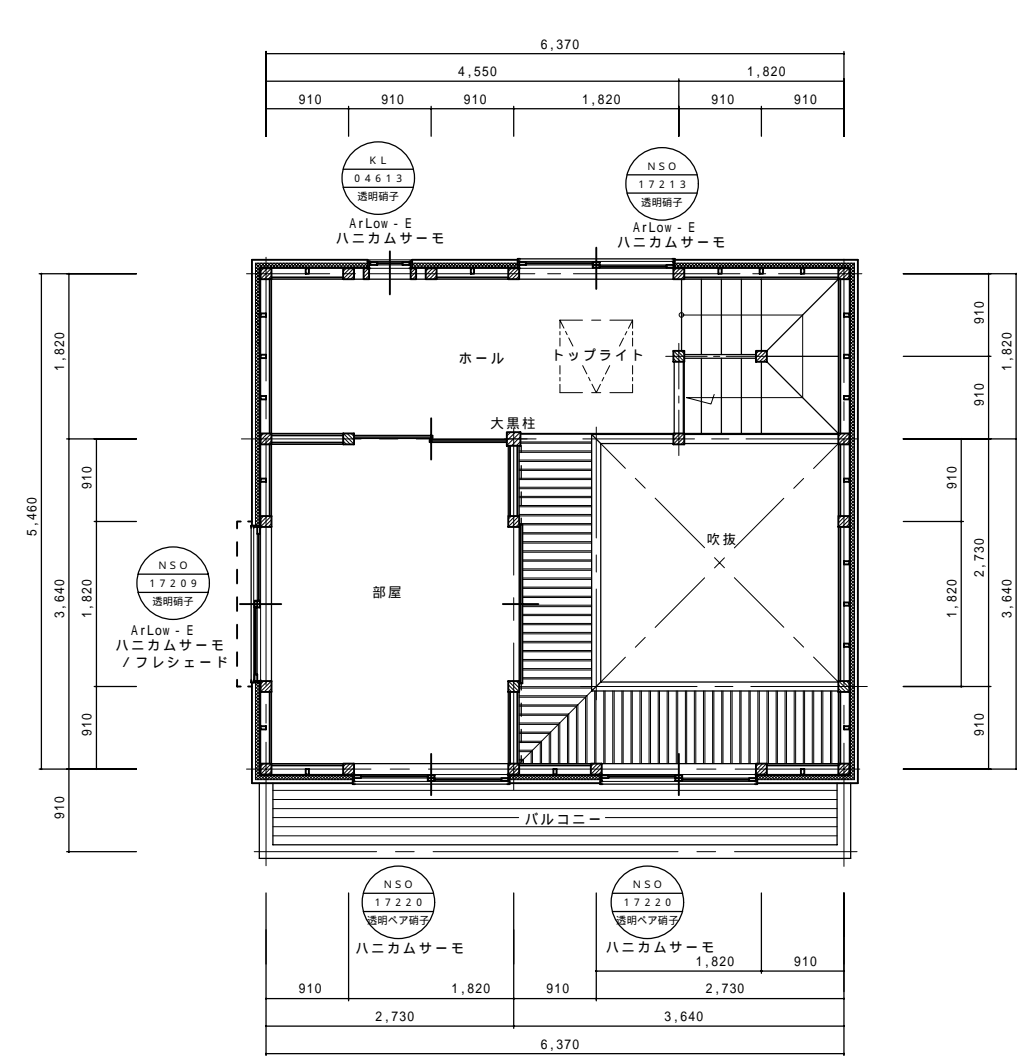
3 F 平面
